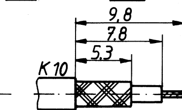
löten solder
