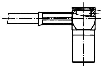
löten solder
