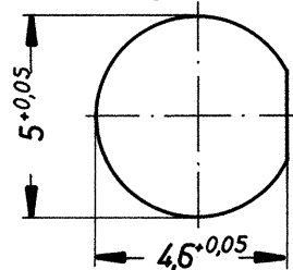
Montagedurchbruch
