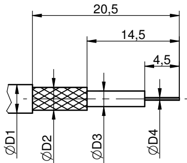
Kabelzuschnitt Ⓞ Stripping dimension
